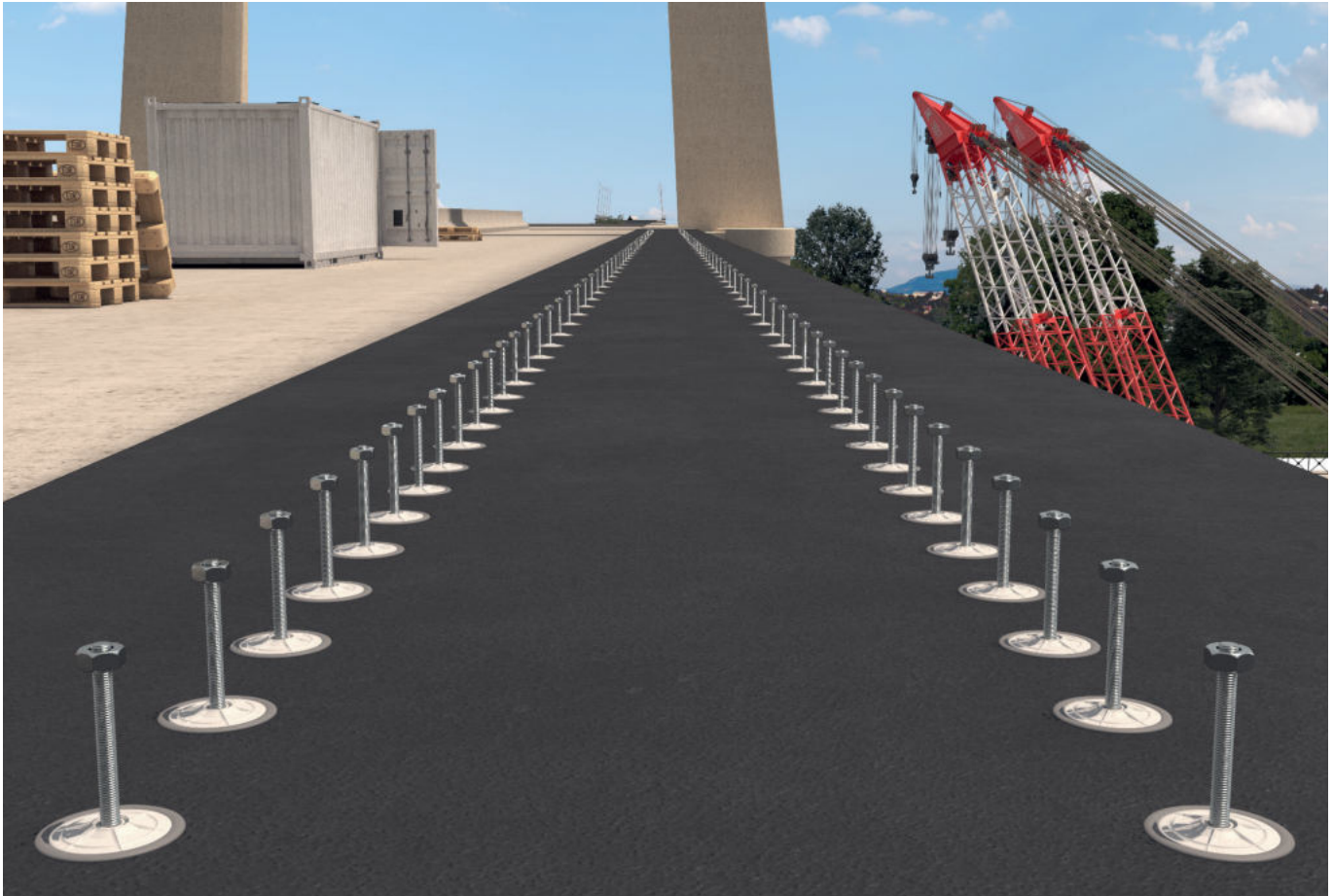
Brückenkappenanker FCC-B
