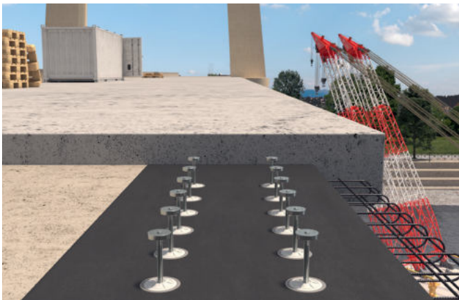
FCC-B Detailsicht
