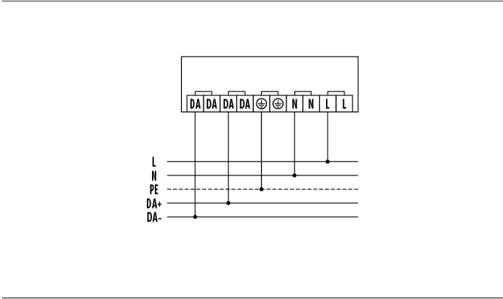
Standardbetrieb DALI/DALI-2.
