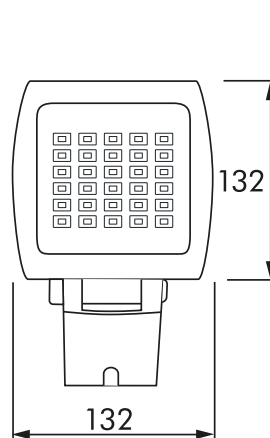
Bemaßung 92702
