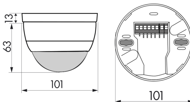
Bemaßung 92440
