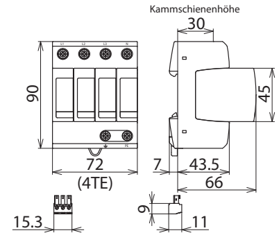
Maßbild DG M TT 385 FM
