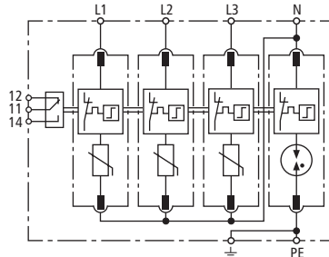
Prinzip Schaltbild DG M TT 385 FM
