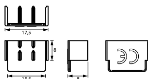
Maßzeichnung Gruppenansicht
