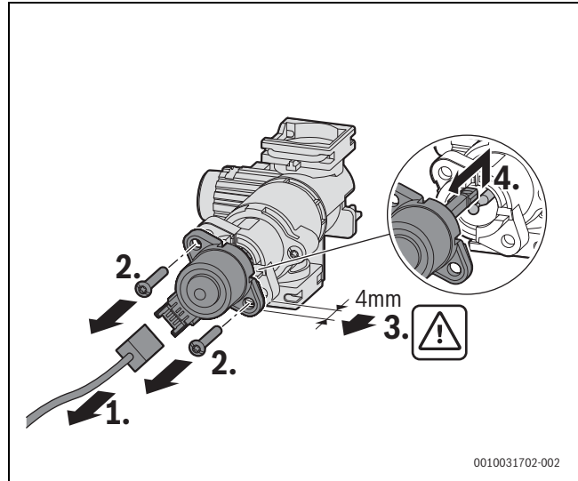
Bild 90 Motor am 3-Wege-Ventil ausbauen (Variante mit Schrauben)
