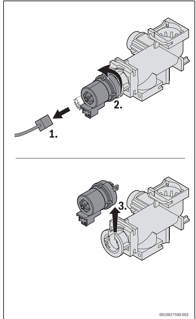
Bild 88 Motor am 3-Wege-Ventil ausbauen (Variante ohne Schrauben)
