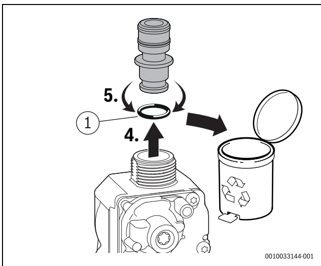
Bild 75 Gasdrossel abnehmen
