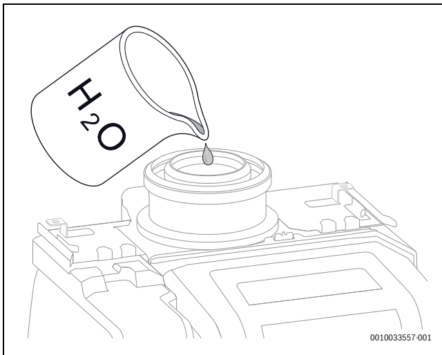
Bild 39 Kondensatsiphon mit Wasser füllen
