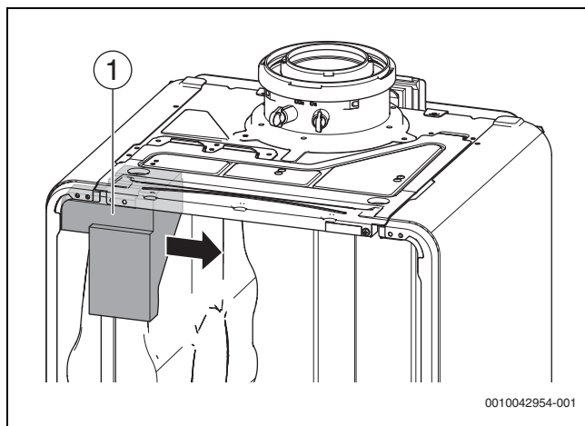
Bild 36 Stützschaum entfernen
