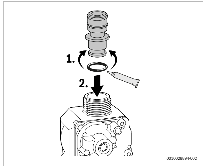
Bild 80 Gasdrossel einsetzen
