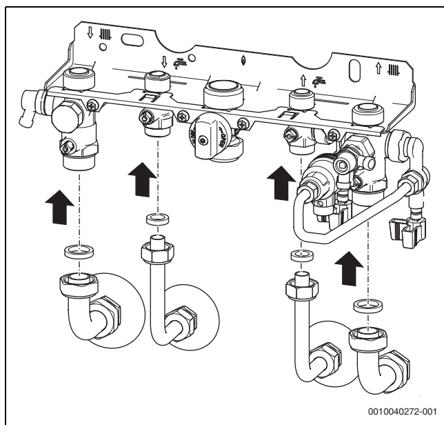
Bild 35 Rohre mit Dichtungen an Montageanschlussplatte (Zubehör) montieren
