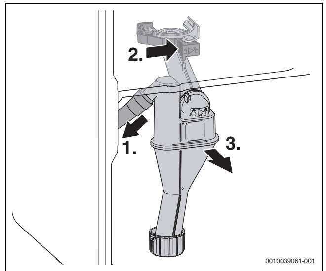
Bild 83 Kondensatsiphon ausbauen
