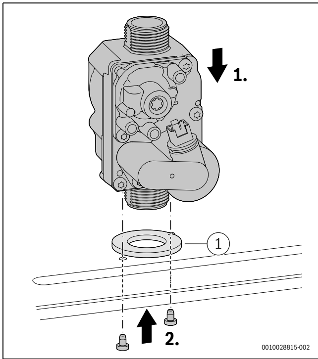
Bild 78 Gasarmatur einbauen
