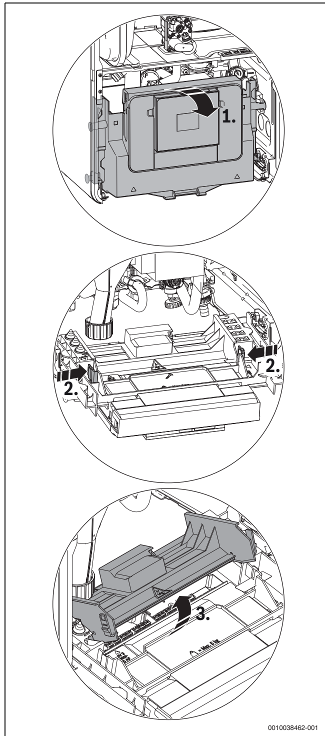
Bild 43 Abdeckung aufklappen
