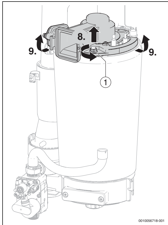
Bild 58 Brennerdeckel mit Gebläse und Mischeinrichtung abnehmen
