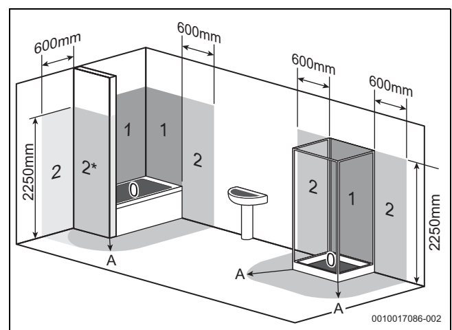
Bild 32 Schutzbereiche (Beispieldarstellung)
