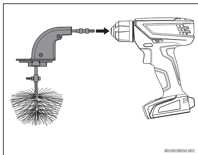
Bild 63 Bürste mit Akku-Schrauber verbinden
