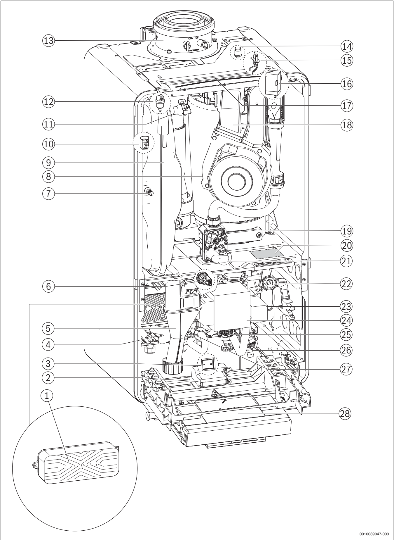
Bild 6 Produktübersicht Kombigerät
