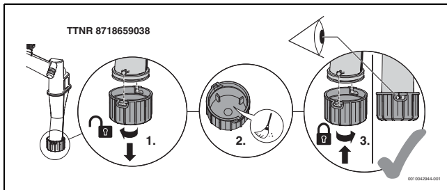
Bild 84 Schmutzfänger reinigen
