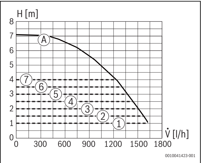
Bild 92 Pumpenkennfelder und Pumpenkennlinien
