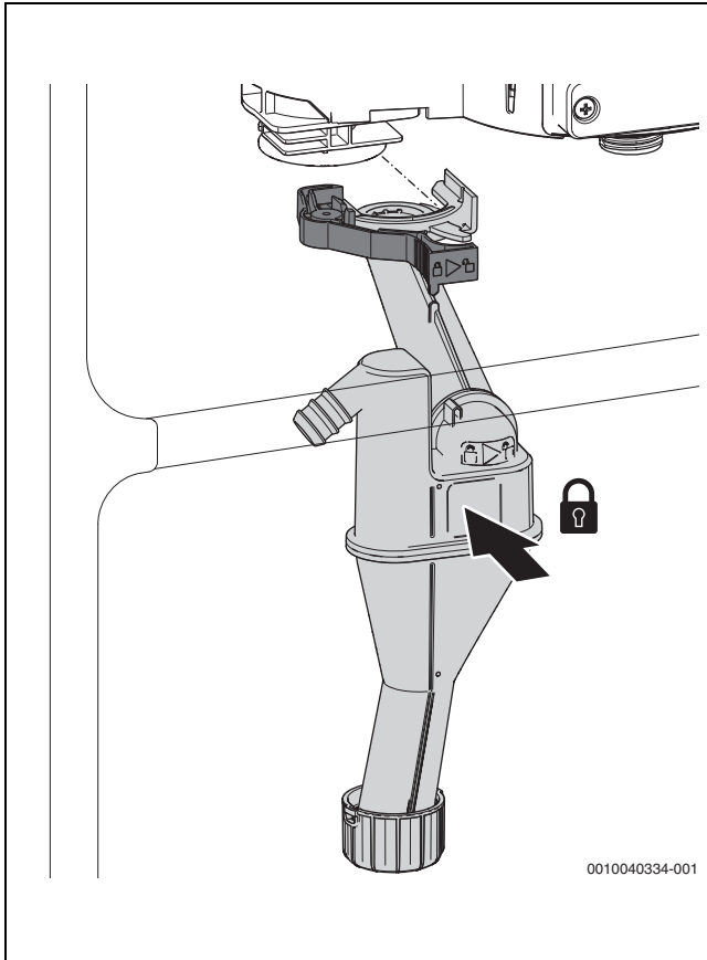
Bild 87 Kondensatsiphon einsetzen
