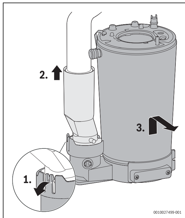
Bild 69 Wärmeblock ausbauen
