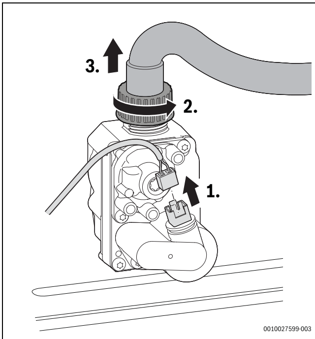
Bild 74 Stecker an der Gasarmatur abziehen und Überwurfmutter mit Gasschlauch abnehmen
