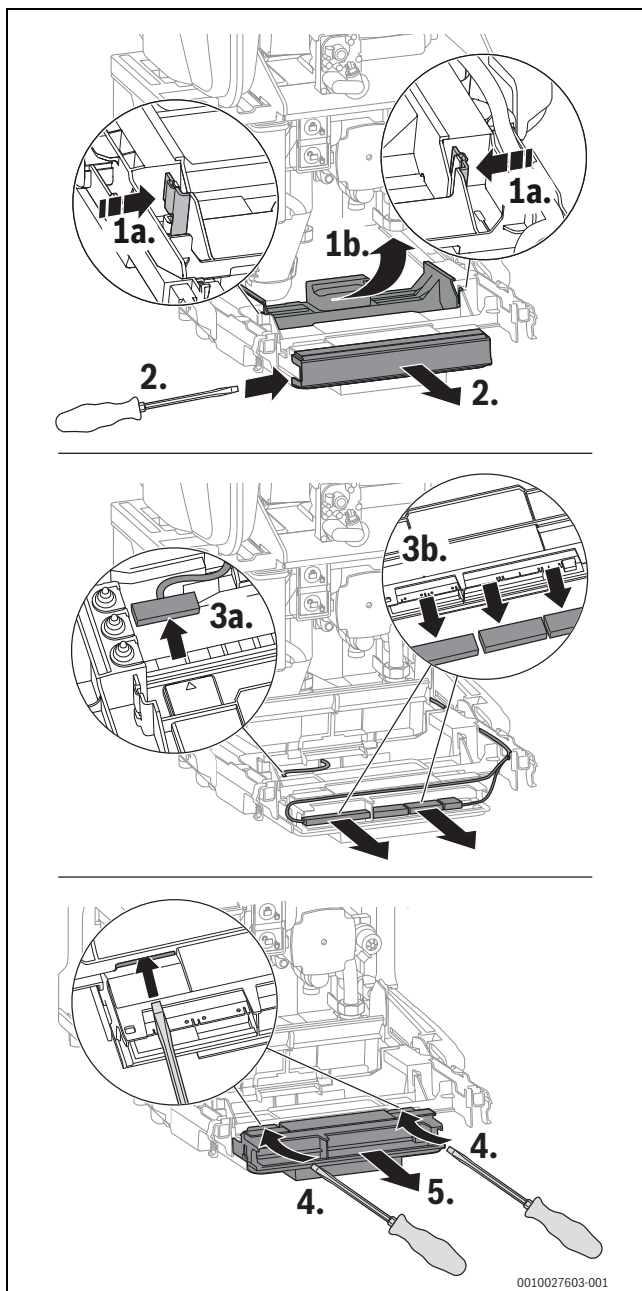
Bild 82 Steuergerät herausnehmen
