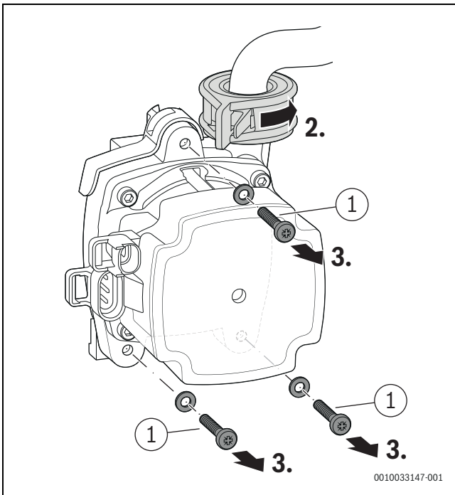
Bild 71 Heizungspumpe entriegeln und Schrauben entfernen
