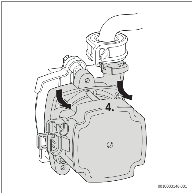
Bild 72 Heizungspumpe abnehmen
