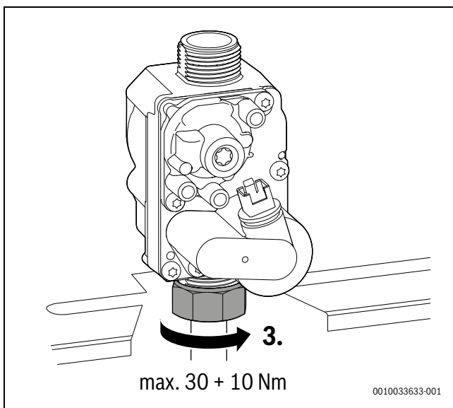
Bild 79 Anzugsdrehmoment beachten
