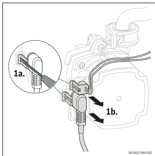
Bild 70 Stecker an der Heizungspumpe abziehen
