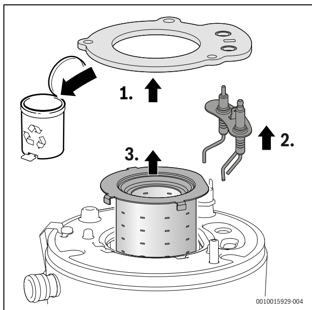
Bild 59 Brenner herausnehmen
