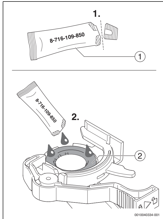
Bild 86 Dichtung fetten
