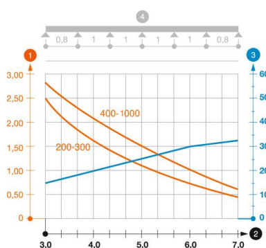
Belastungsdiagramm Weitspannkabelleiter Typ WKLG 110
