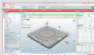
Bemessung und Darstellung der Stahlanschlussplatte nach FE- Methode
