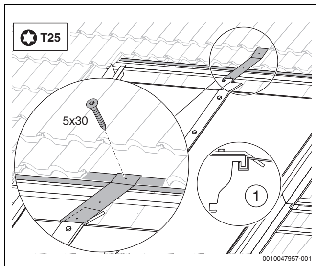
Bild 70 Senkrechte Ausführung
