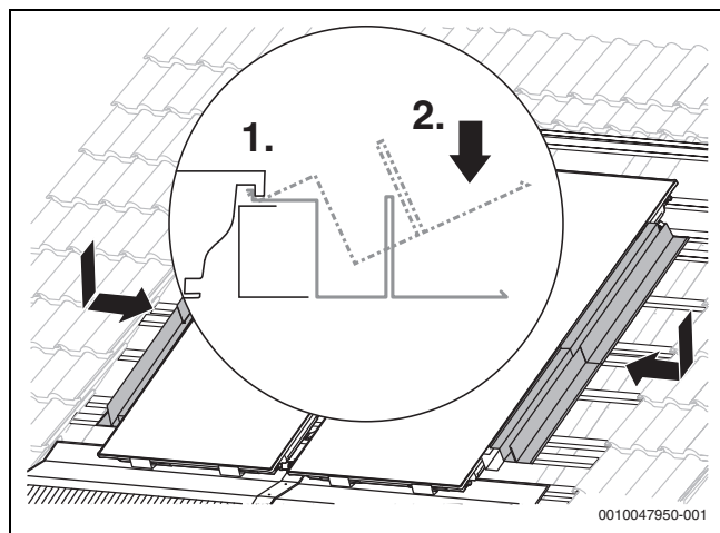
Bild 63 Seitliche Eindeckbleche montieren
