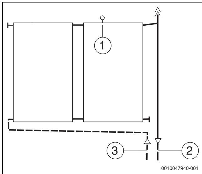
Bild 51 Position des Kolleortemperaturfühlers
