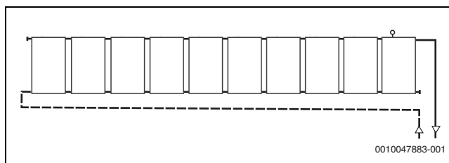
Bild 12 Wechselseitiger Anschluss (1 Reihe)
