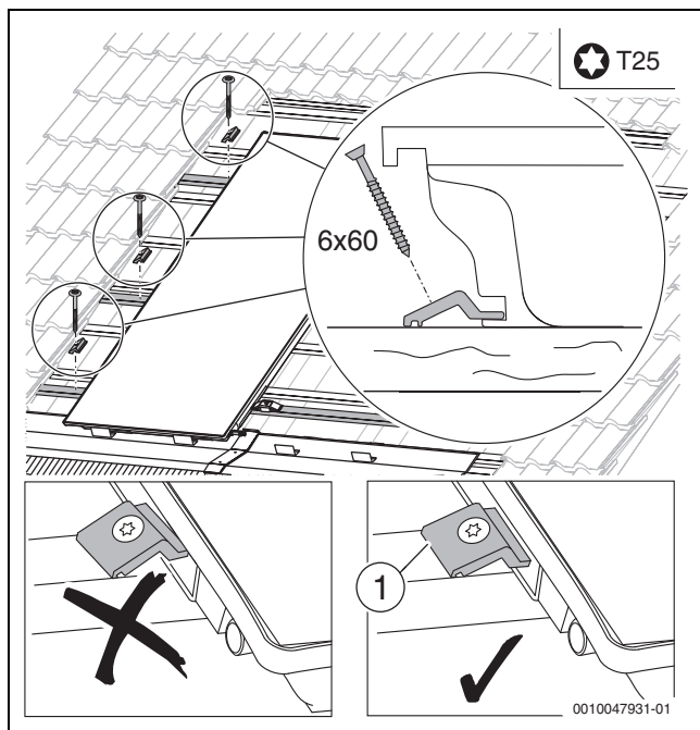
Bild 42 Niederhalter festschrauben
