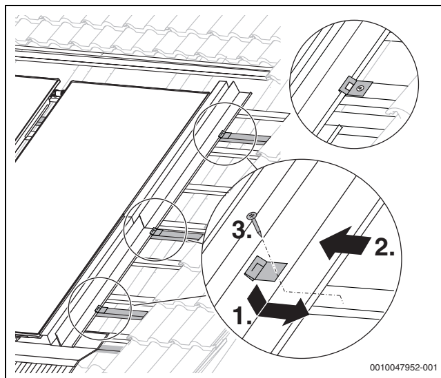
Bild 65 Hafter montieren
