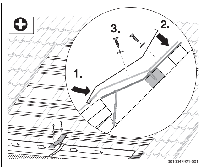
Bild 33 Oberteil montieren
