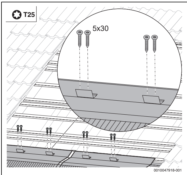
Bild 32 Abrutschsicherungen befestigen
