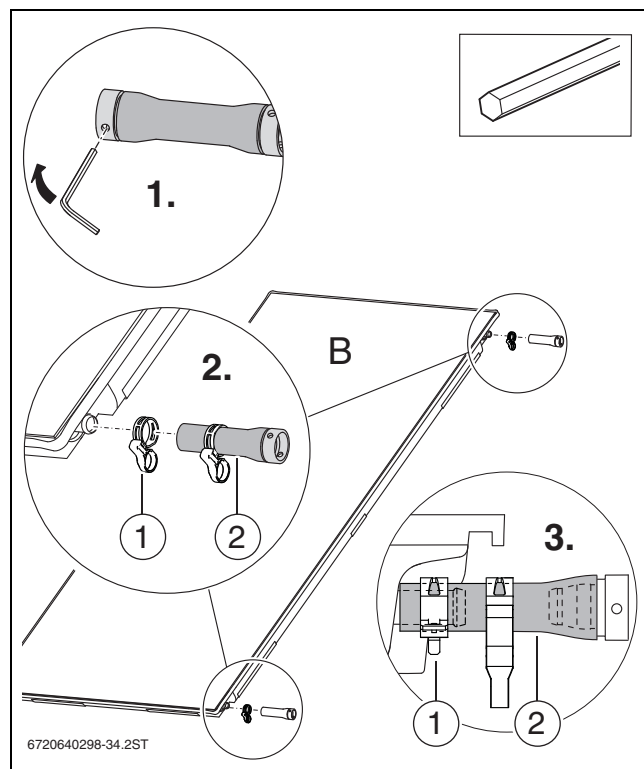
Bild 37 Verbindungs-Set am zweiten Kollektor und alle weiteren montieren
