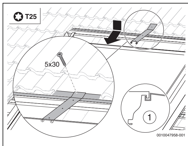
Bild 71 Waagerechte Ausführung
