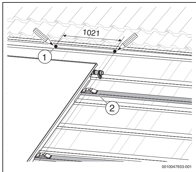
Bild 44 Montageposition des oberen Verbinders bei waagerechten Kollektoren
