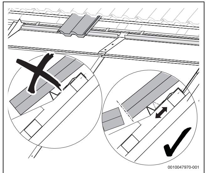
Bild 82 Dachziegelaufgabe positionieren
