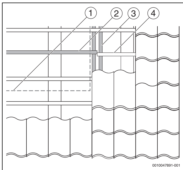
Bild 23 Dachlatte versetzen
