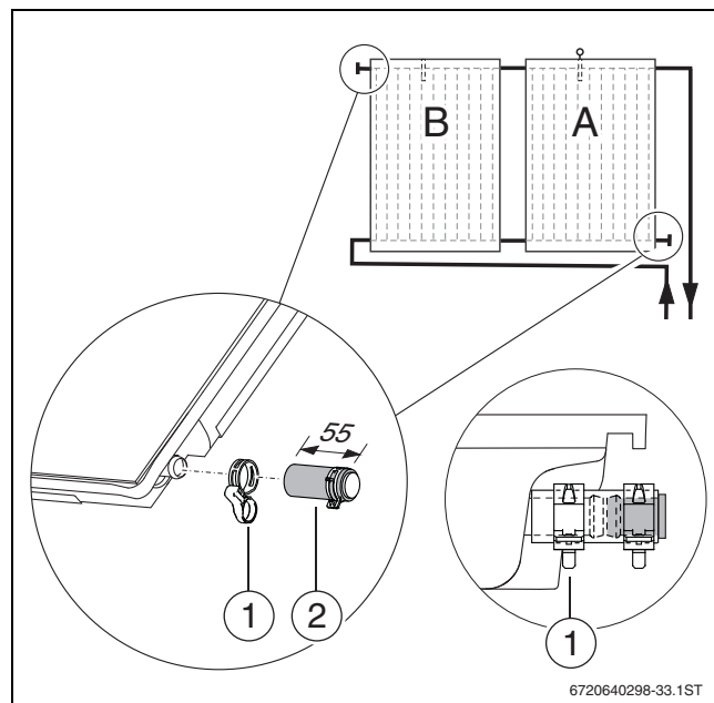
Bild 36 Stopfen montieren
