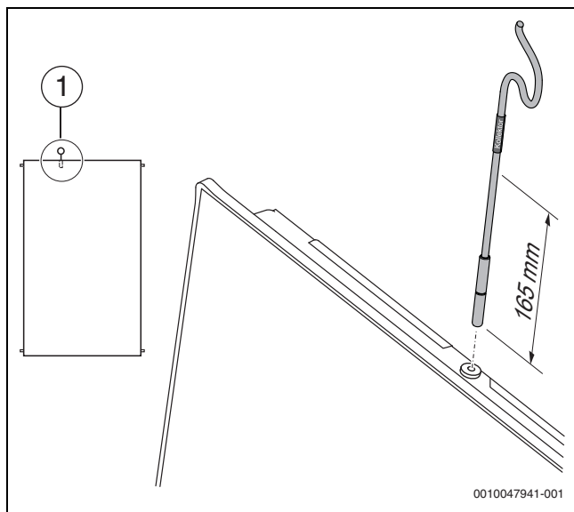
Bild 52 Kolleortemperaturfühler montieren
