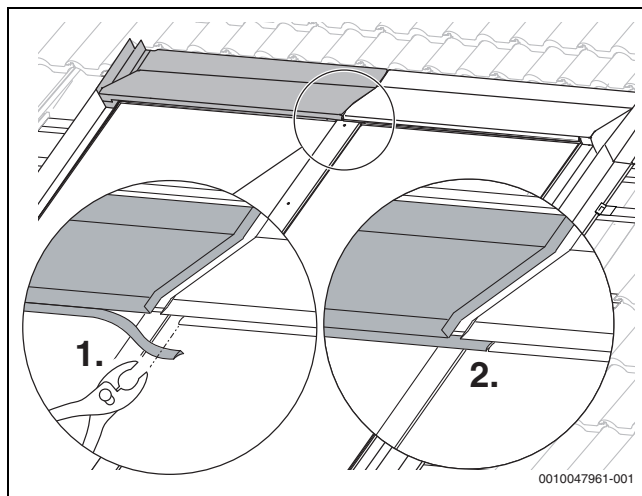
Bild 74 Dichtlippe anpassen
