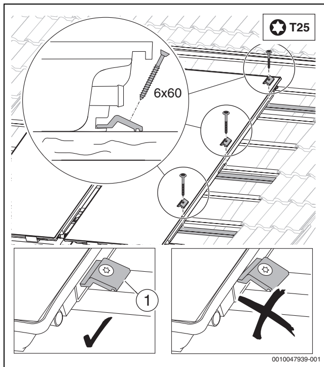
Bild 50 Niederhalter festschrauben
