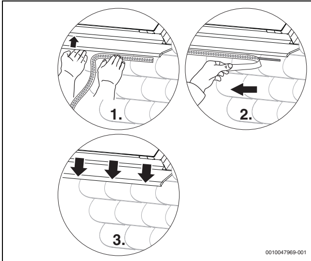
Bild 81 Unterer Eindeckblech auf Eindeckung kleben
