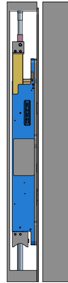
Detail Y 1:5 IQ AUT
