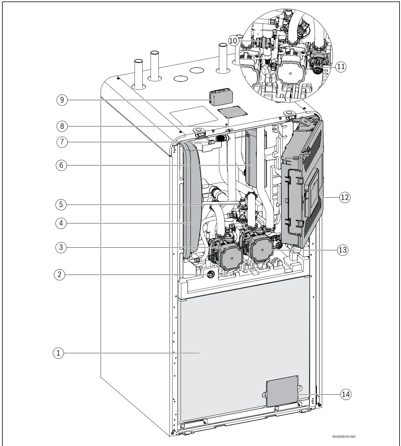
Bild 5 Inneneinheit
