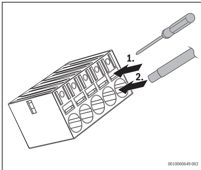
Bild 33 Kabelinstallation
