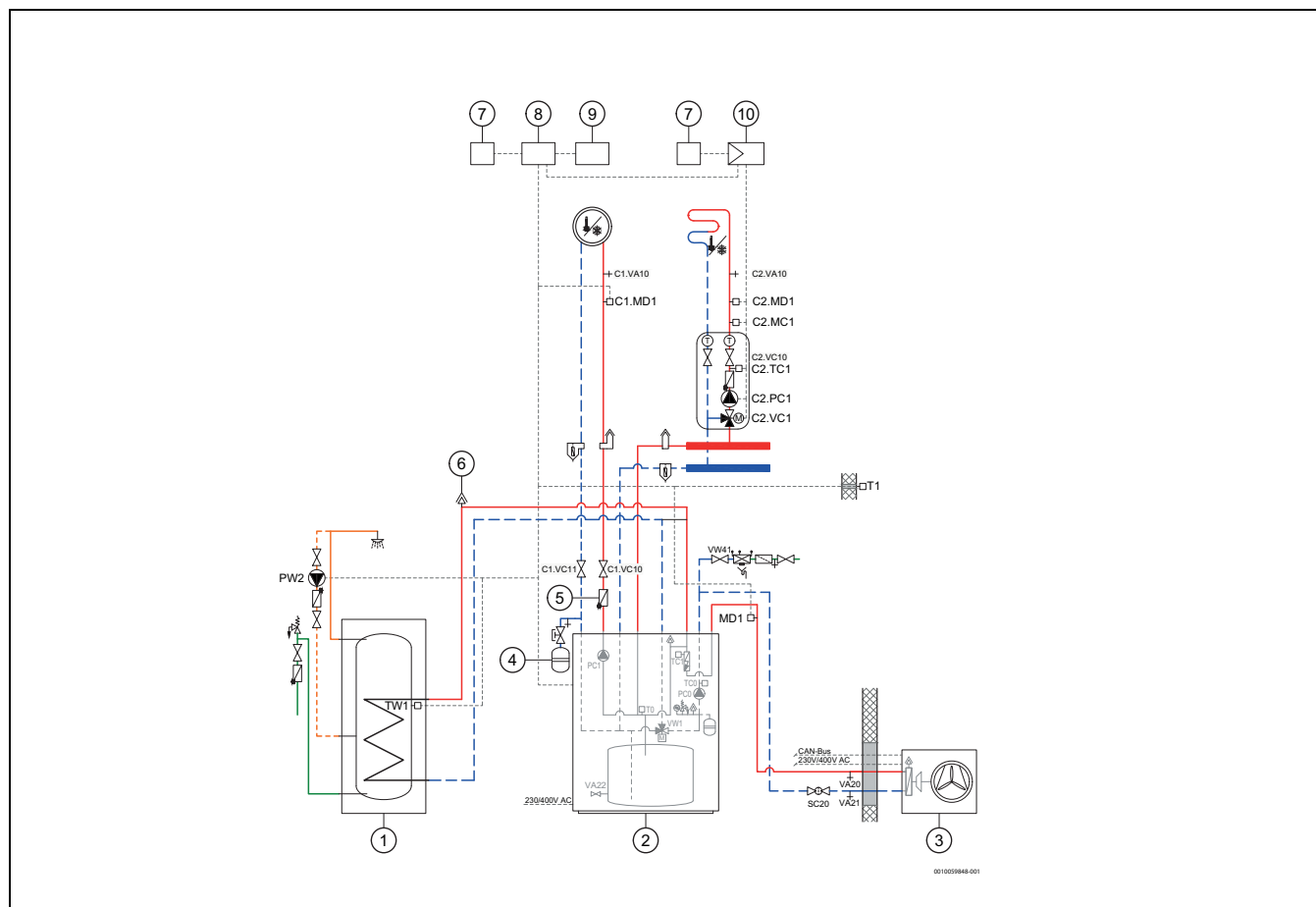
Bild 47 Anlagen mit Außeneinheit, Inneneinheit mit integriertem elektrischem Zuheizter und Pufferspeicher und einem ungemischten und einem gemischten Heizkreis
