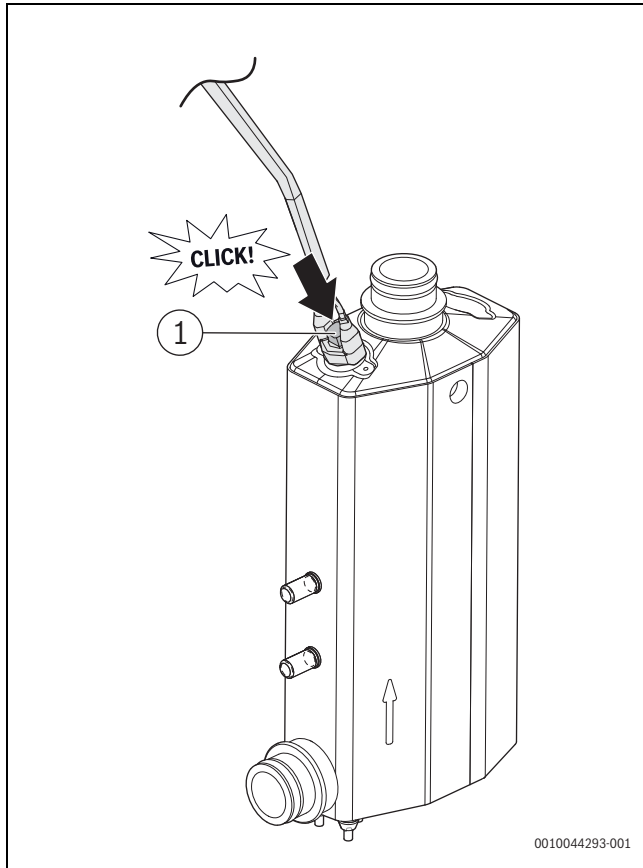
Bild 43 Elektrischer Zuheizer
