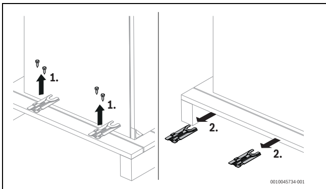
Bild 8 Transportsicherungen entfernen
