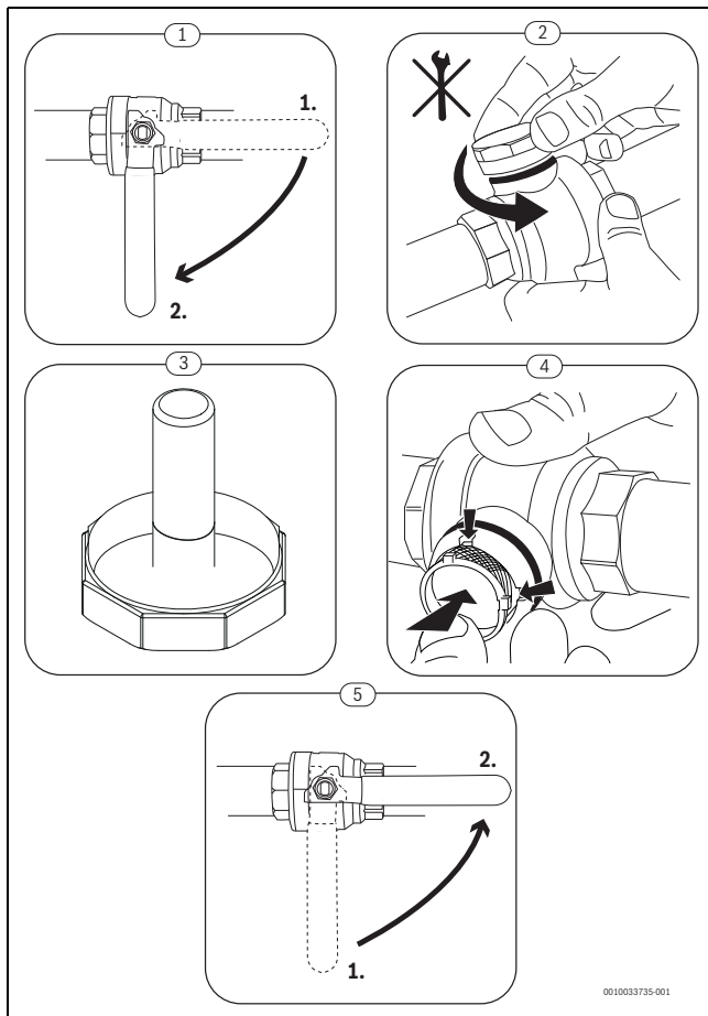
Bild 45 Filterreinigung
