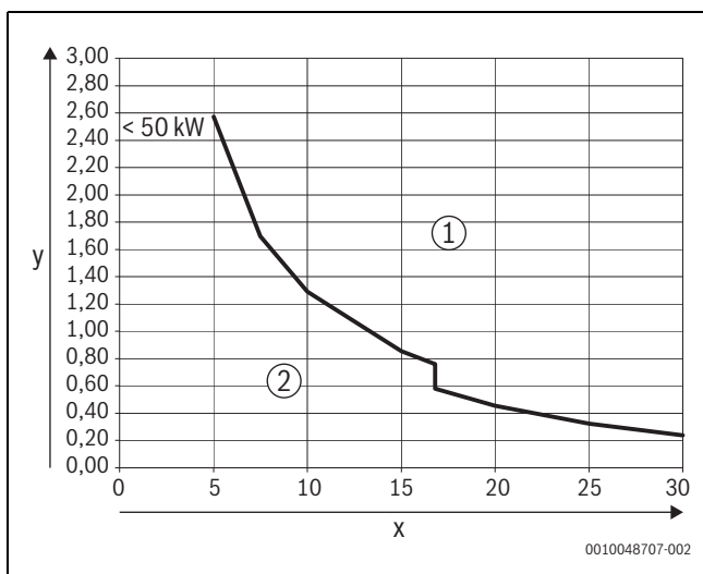
Bild 6 Wärmezeuger < 50 kW - 100 kW
