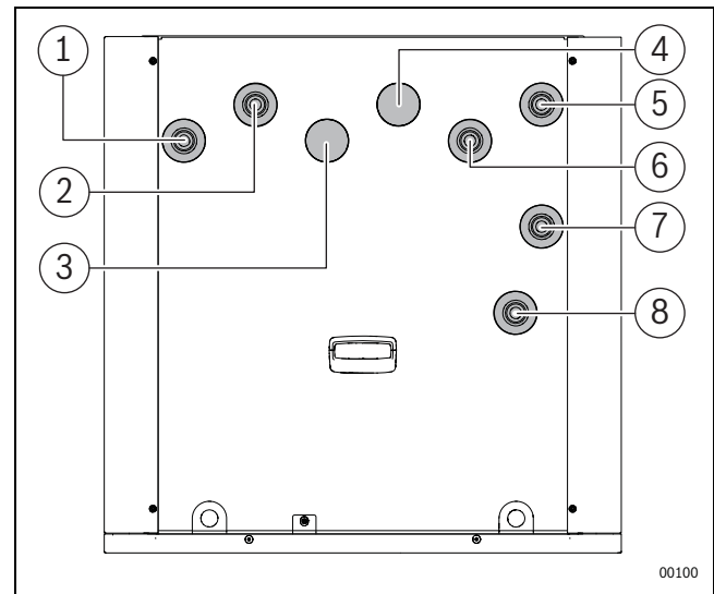
Bild 15 Hydraulische Anschlüsse
