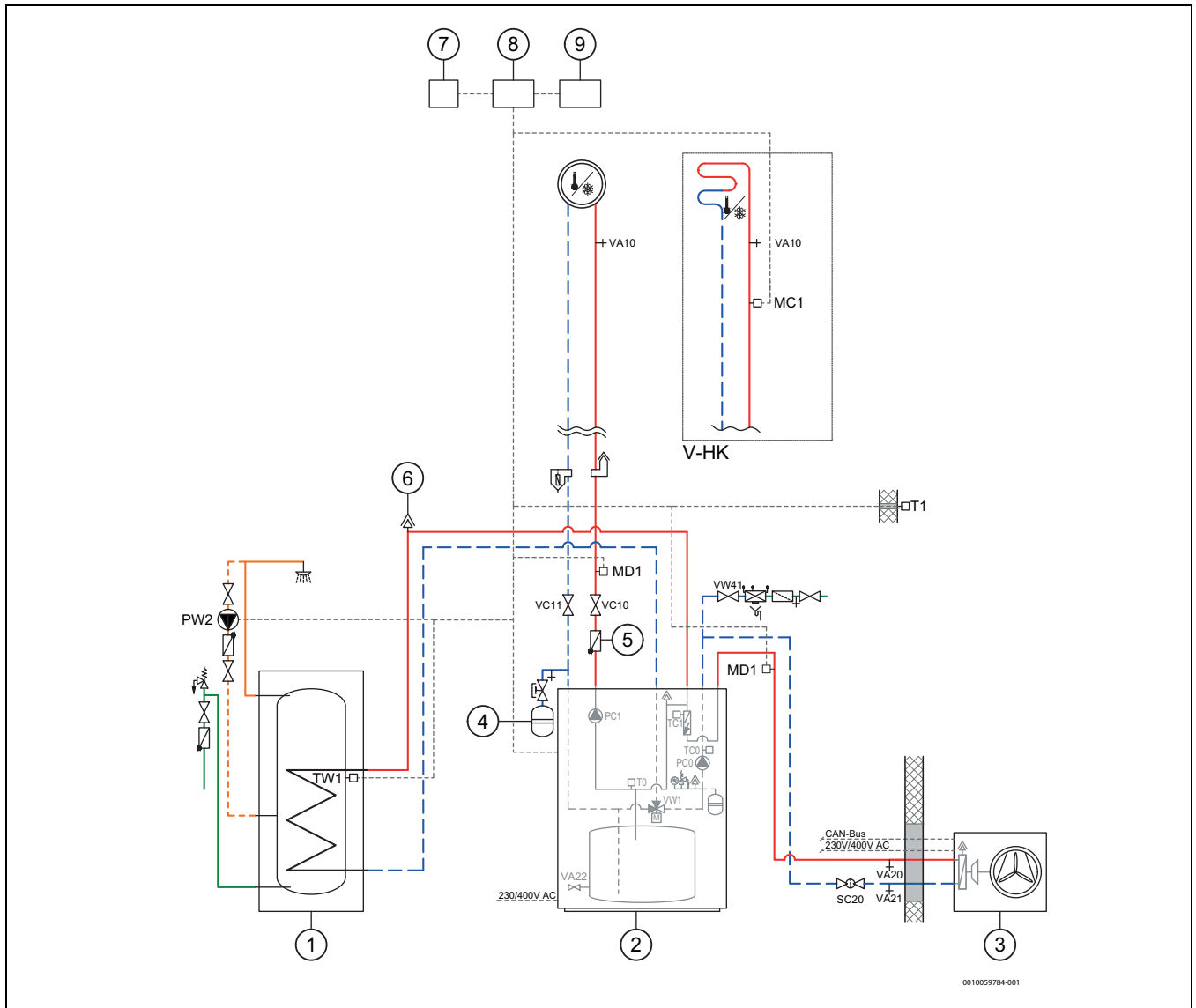
Bild 46 Anlage mit Außeneinheit, Inneneinheit mit integriertem elektrischem Zuheizter und Pufferspeicher und einem ungemischtem Heizkreis
