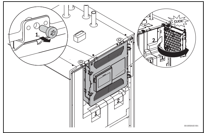
Bild 44 Klemmenkasten
