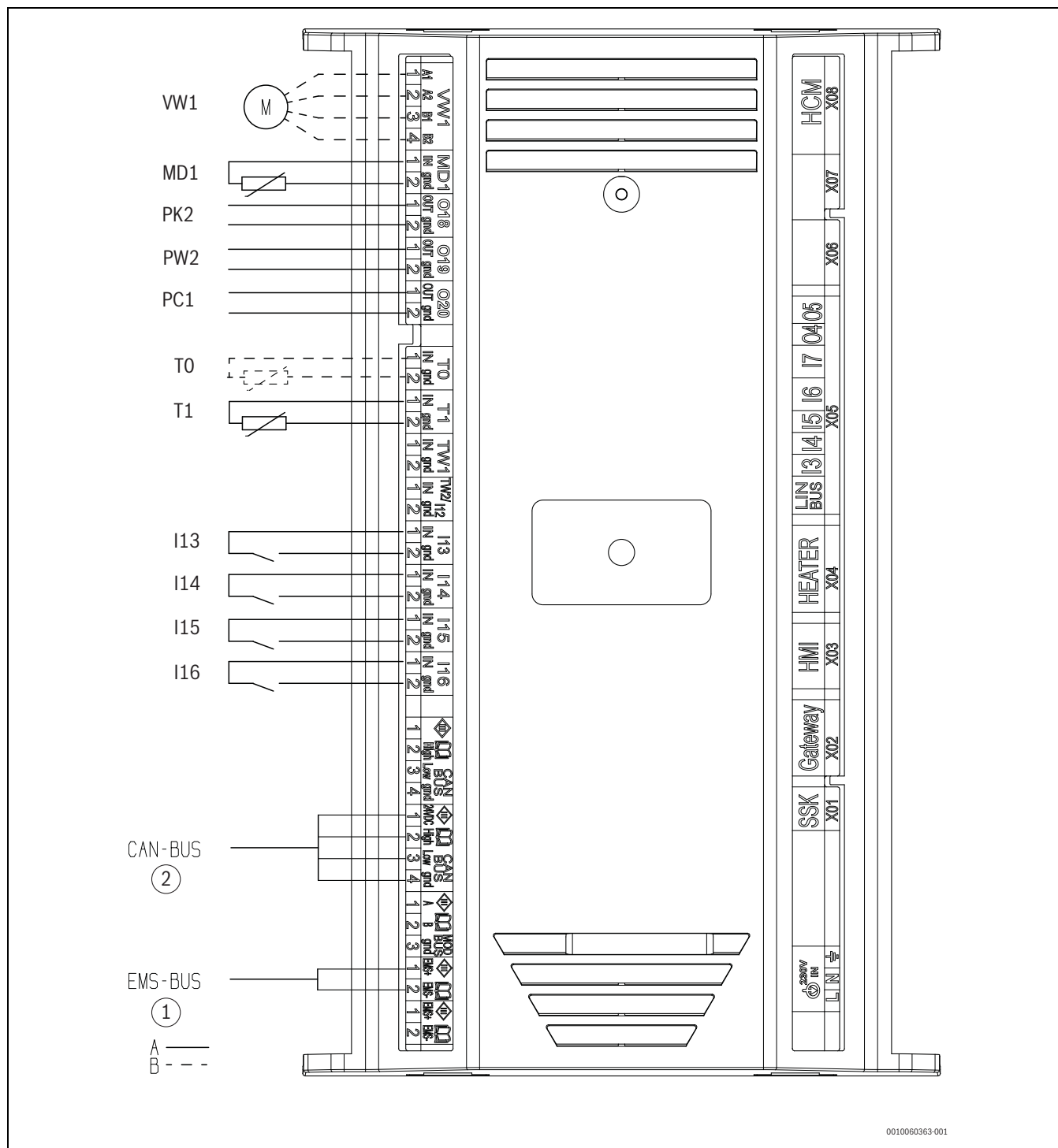
Bild 41 Anschlüsse XCU-THH
