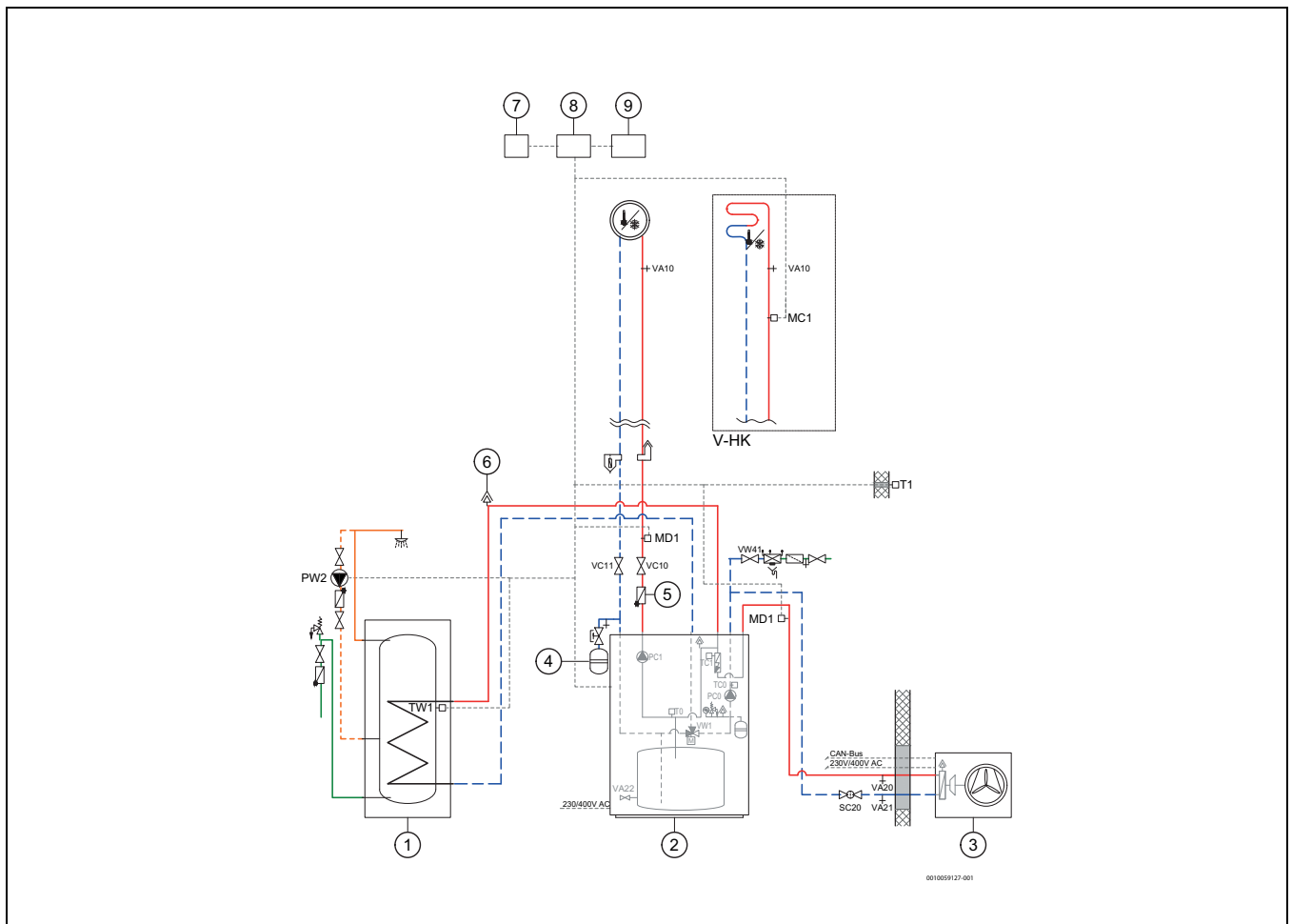
Bild 21 Anlagenlösung mit Außeneinheit, Inneneinheit mit integriertem elektrischem Zuheizung und Pufferspeicher und einem ungemischtem Heizkreis
