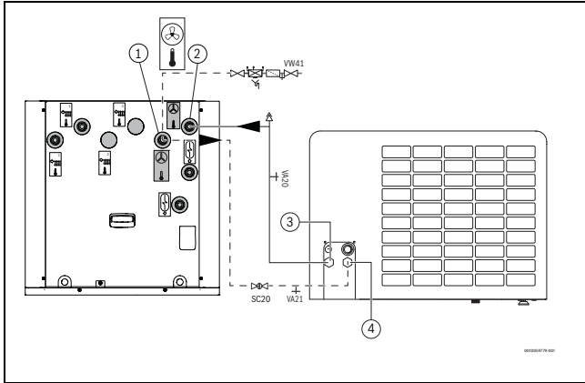
Bild 16 Außeneinheit anschließen
