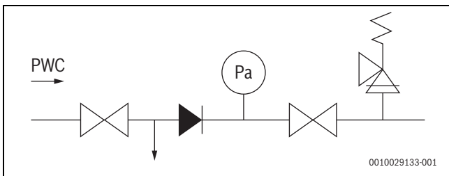
Bild 17 Beispiel: Sicherheitsgruppe für Expansionswasser nach EN 1488
