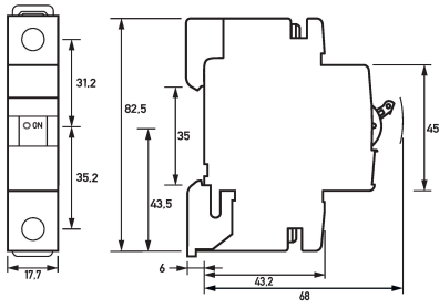
Maßzeichnung Gruppenansicht
