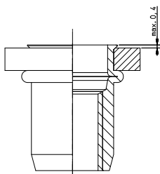
Standard Senkkopf Blindnietmutter in einer glatten Bohrung; Überstand ca. 0,4mm.
